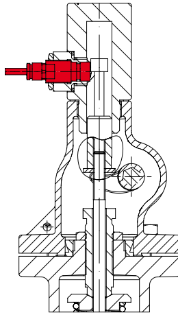
Näherungsschalter
