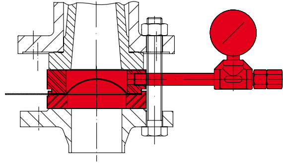
Berstscheibe
